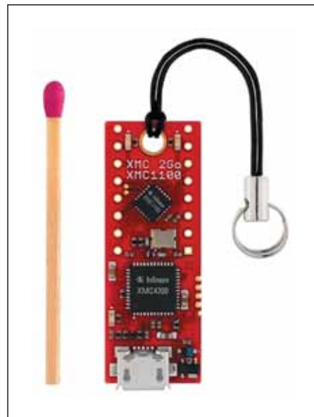
Рис. 1. Оценочная плата XMC2GO с микроконтроллером XMC1100
