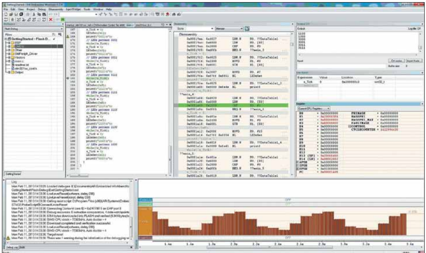
Рис. 1. Внешний вид окна программы EWARM в режиме отладки
