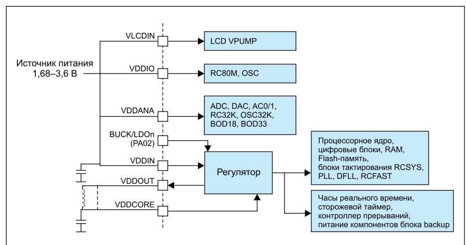
Рис. 1. Схема питания ядра и периферии ATSAM4L
