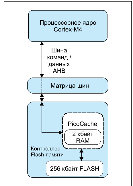
Рис. 3. Считывание команд с использованием PicoCache
